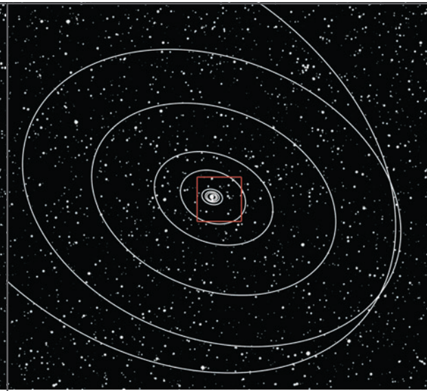
10 15 metri - A 10 miliardi di chilometri di distanza si vede tutta l'area percorsa dai pianeti del Sistema solare, sono evidenziate le orbite dei pianeti esterni (Giove, Saturno, Urano e Nettuno). Plutone, secondo la nuova classificazione dei corpi del Sistema solare, è il primo pianeta nano.
